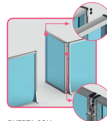
PUERTA CON APERTURA A 90° Y 180°: Puerta abisagrada para apertura de hasta 180° con topes protectores y cerradura de agarre.
