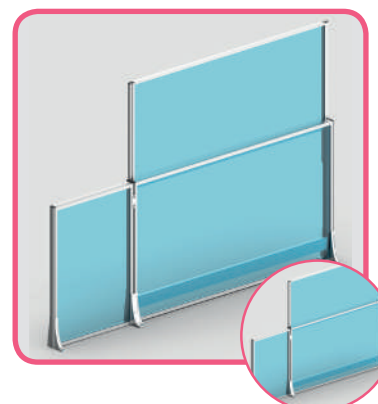
COMBINACIÓN ENTRE VIDRIO FIJO/MÓVIL: Combina entre sí las opciones de vidrio fijo o móvil enrasado por fuera o por dentro.
